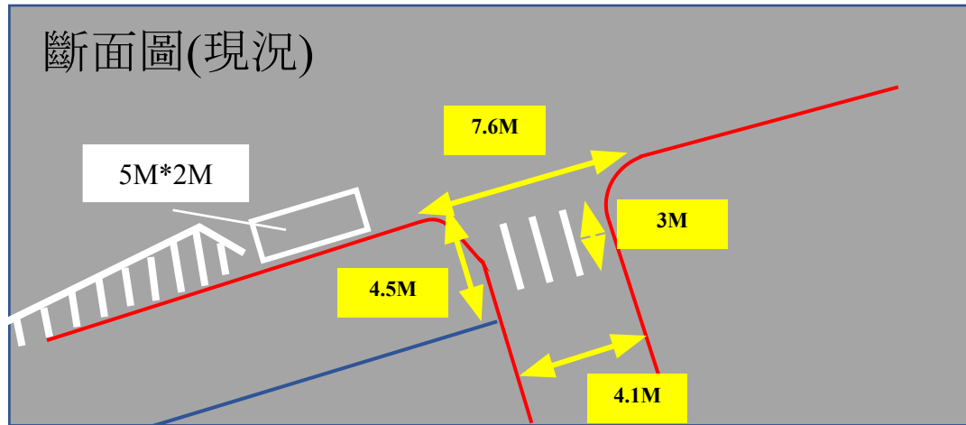
斷面圖(待轉格調整)
